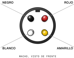
El reparto de contactos de la versión macho
