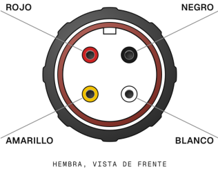
El reparto de contactos de la versión hembra
